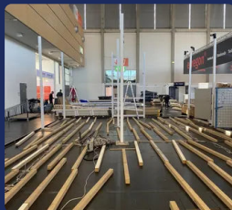
Messestand in Holzrahmenbauweise
